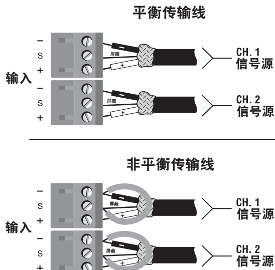
图 2.5 输入接头 Phoenix 型接线，平衡接口（上）和非平衡接口（下）
