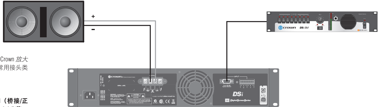
图 2.10 桥接单声道模式接线
