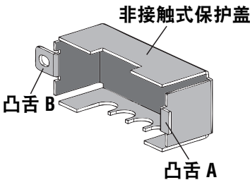
图 2.8 非接触式保护盖内部
