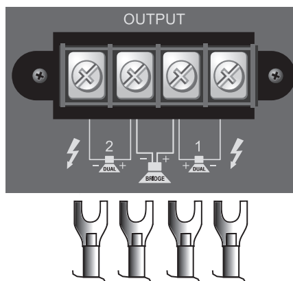
图 2.6 绝缘带输出接线
