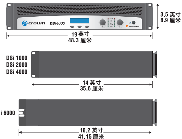
图 2.1 尺寸
