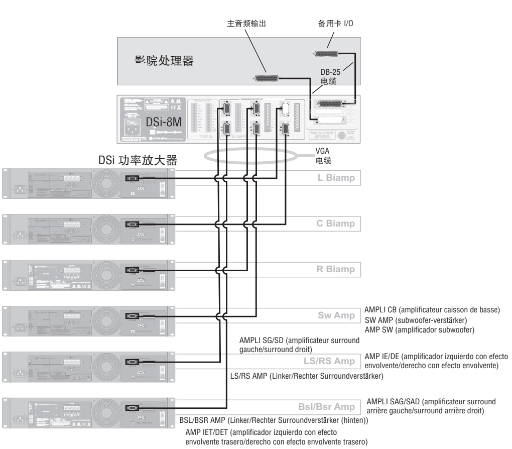
图 2.3 通过 HD-15 接口 将 DSi 功率放大器连接至 DSi-8M 监控面板
